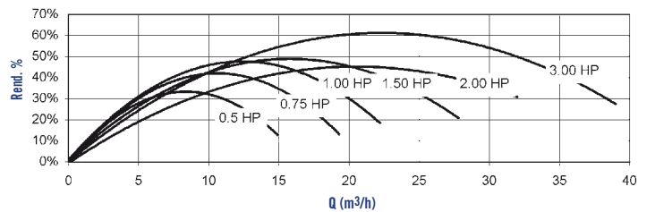
Curvas de rendimiento Performance curve
