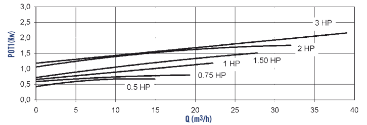
Curvas de Potencia-Caudal Power-Flow Curves
